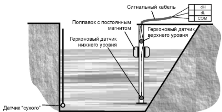
Дренаж с использованием поплавкового датчика уровня
