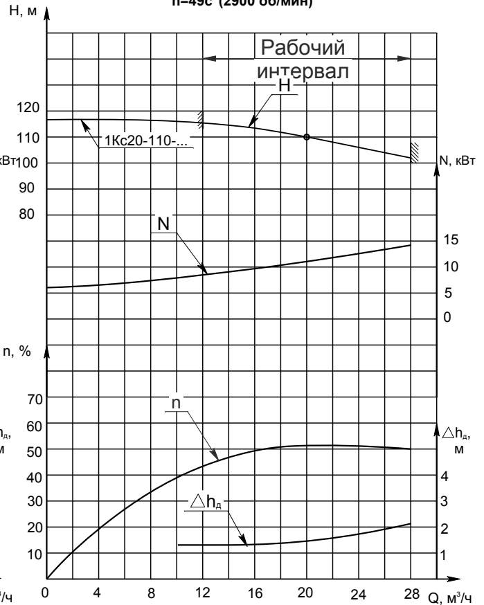
Продолжение приложения А Характеристика насоса 1Кс20-110-... Жидкость- вода \rho=1000 \text{ кг/м}^3 n=49\text{с}^{-1} (2900 об/мин)
