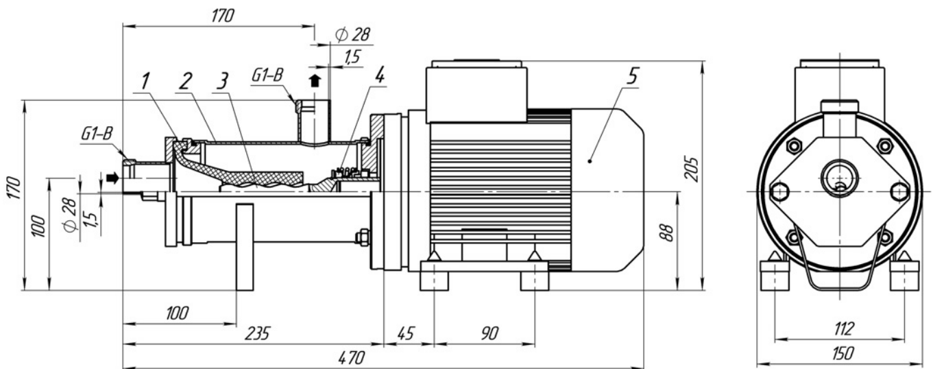
1 – Обойма; 2 – Корпус насоса; 3 – Винт рабочий; 4 – Торцовое уплотнение; 5 – Электродвигатель; 6 – Опора
