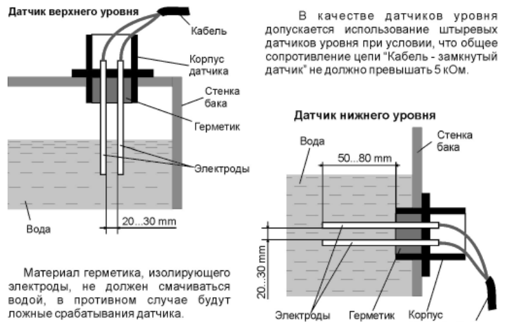
Дренаж с использованием штыревых датчиков уровня
